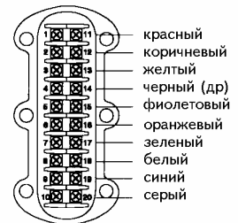
Клеммы модели 3700
